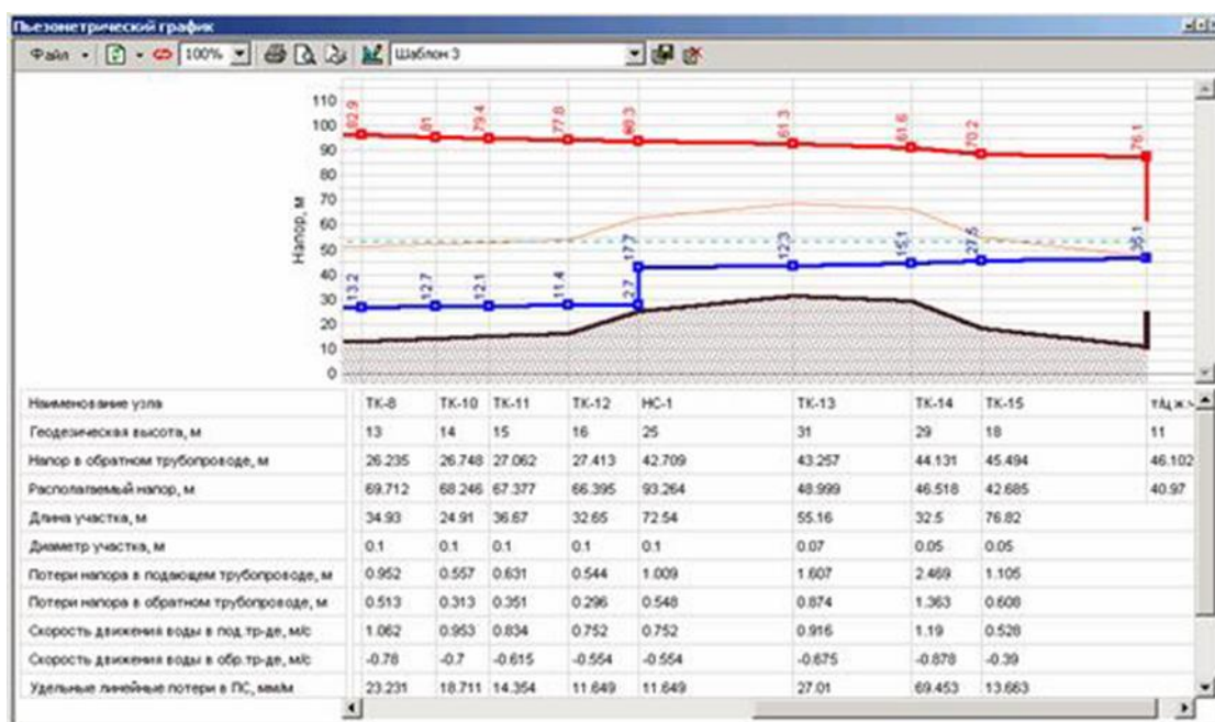
Рисунок 2.23 - Пьезометрический график
