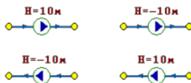
Рисунок 2.14 - Насосная станция
