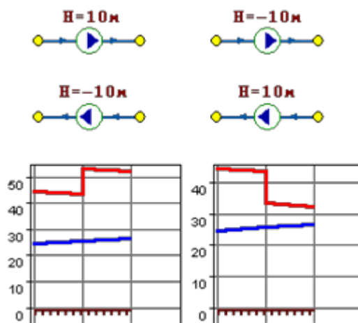
Рисунок 2.15 - Пьезометрические графики
