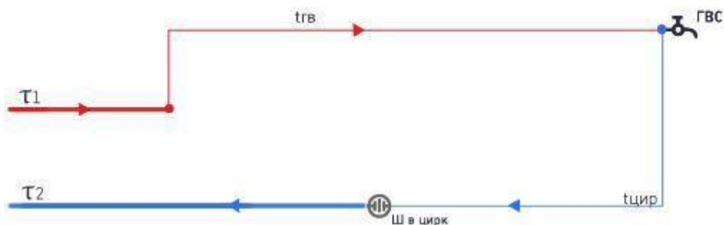
Рисунок 13.4 - Схемы №26 «Потребитель с открытым водоразбором и циркуляционной линией»
