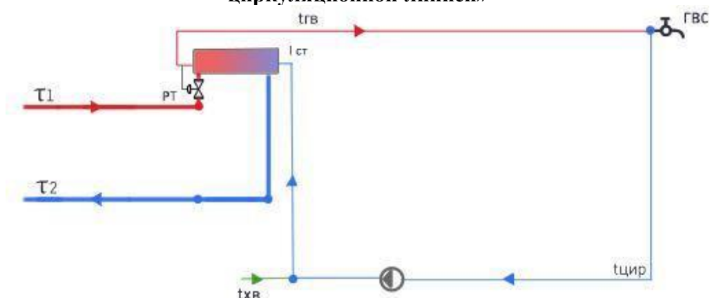
Рисунок 13.5 - Схема №27 «Потребитель с подогревателями ГВС»
