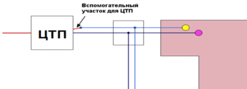
Рисунок 2.5 - Подключение трубопровода ГВС
